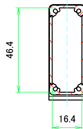
A-A (1:1.5)
