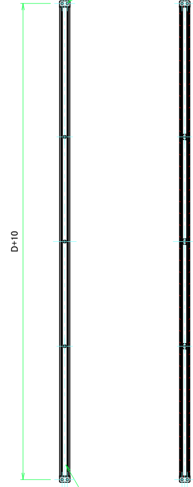
D-D (1:5)
