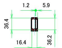
A-A (1:5)
