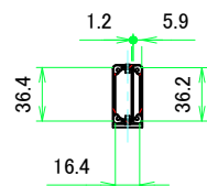
A-A (1:4)
