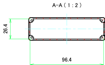
A-A (1:2)
