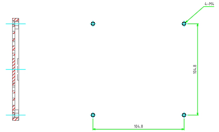
取付穴寸法
