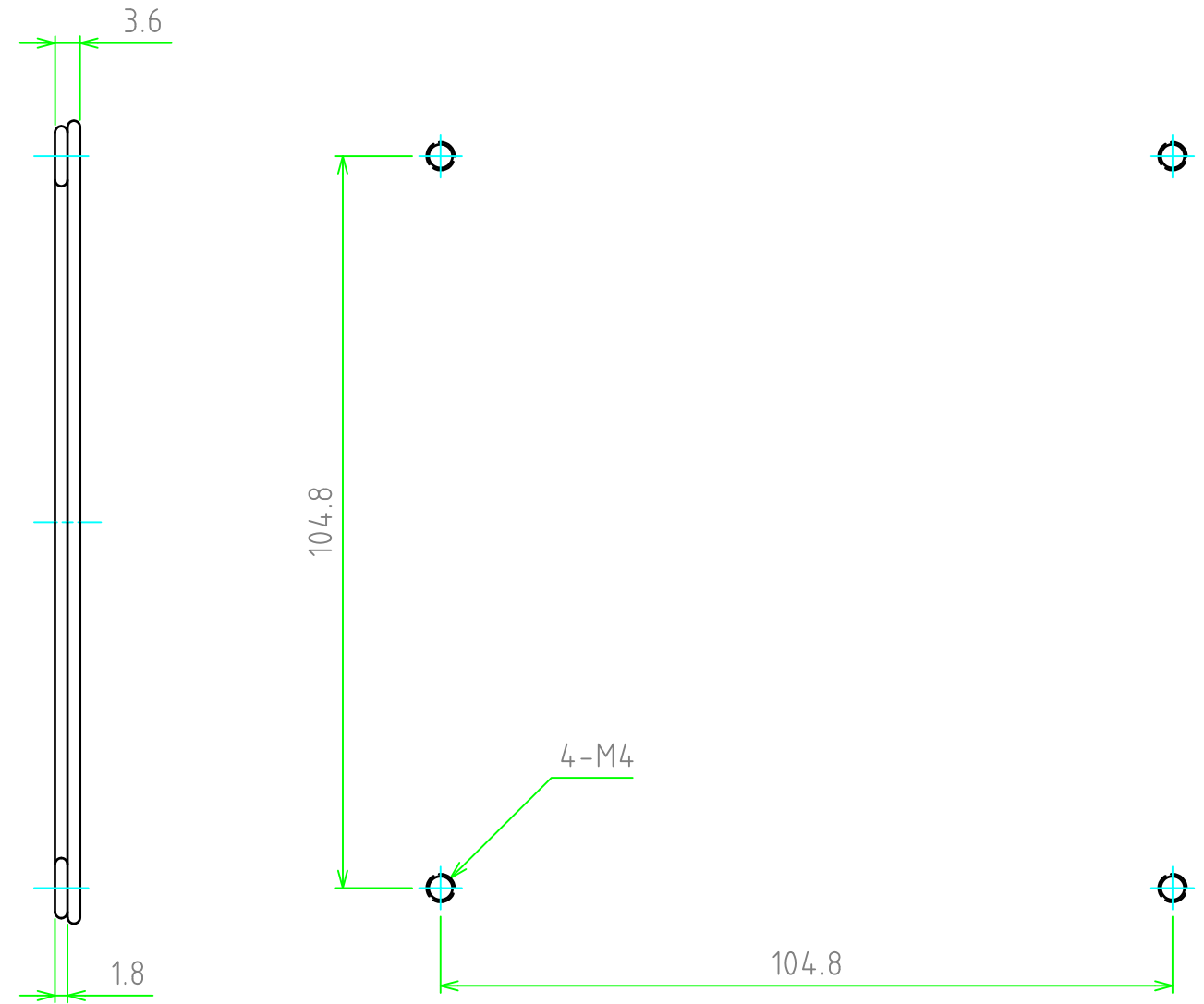
取付穴寸法
