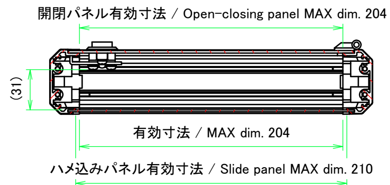
A-A (1:3)
