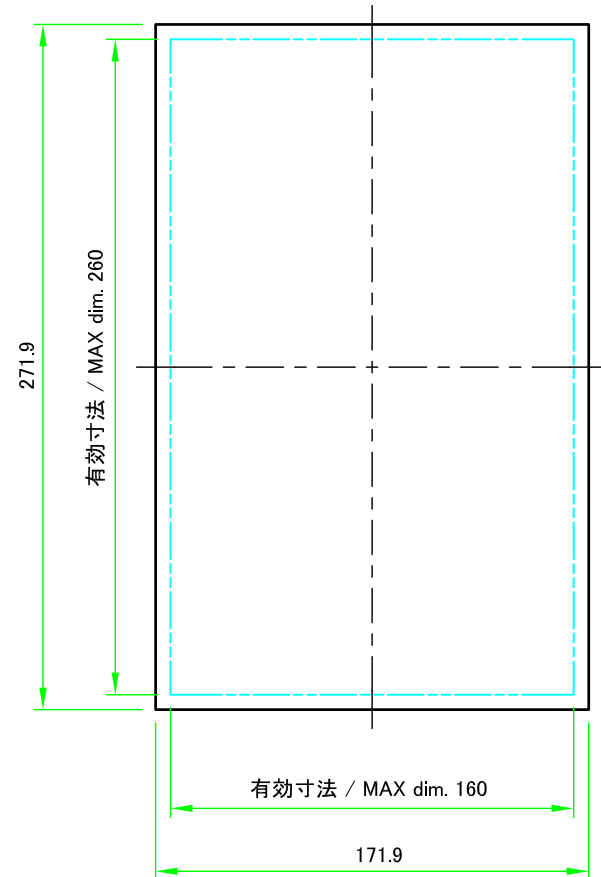
パネル裏面/Panel Frontside
