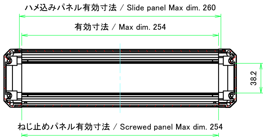
A-A (1:3)
