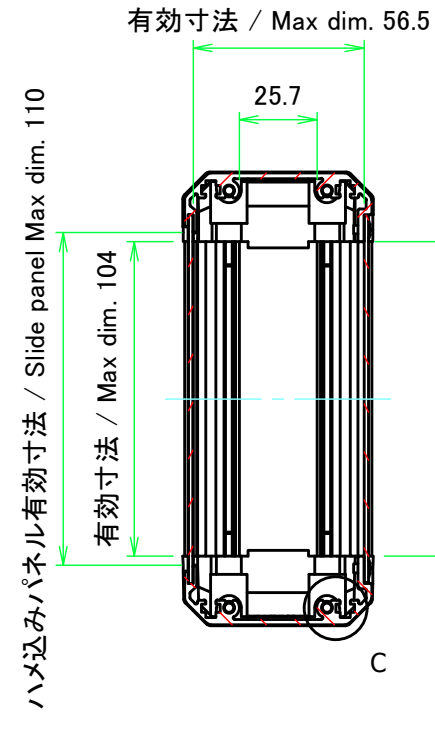
フレーム4側 / Frame4 side
