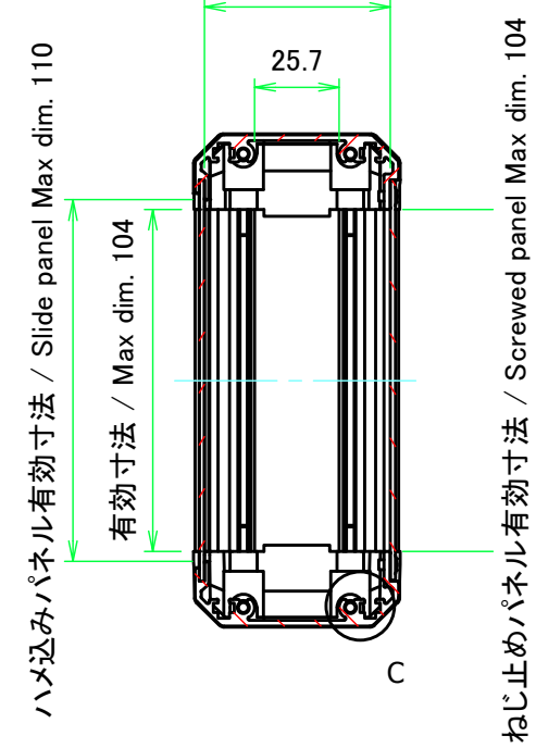
有効寸法 / Max dim. 56.5
