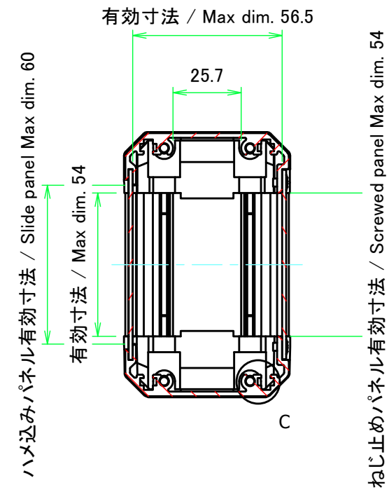
B-B (1:2)
