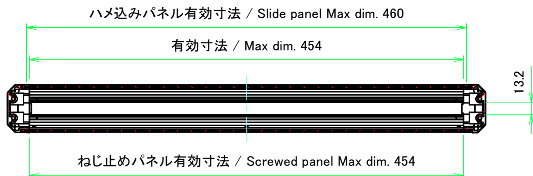
A-A (1:4)
