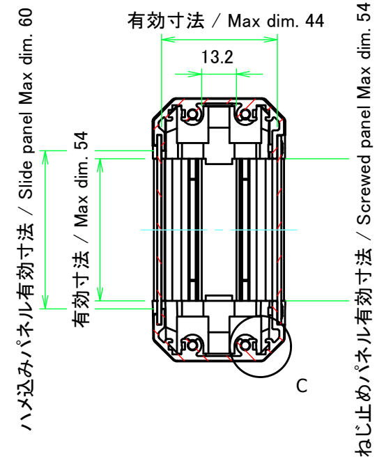
B-B (1:2)
