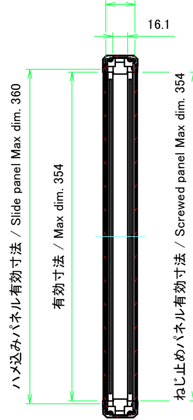
有効寸法 / Max dim. 31.5
