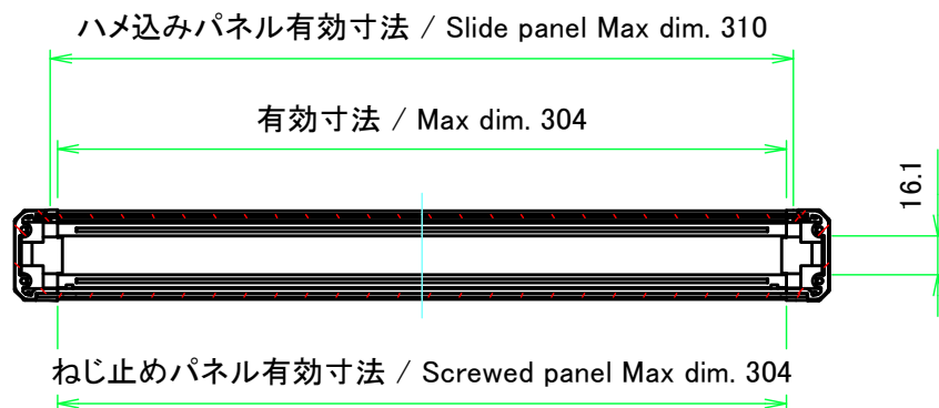
A-A (1:3.5)
