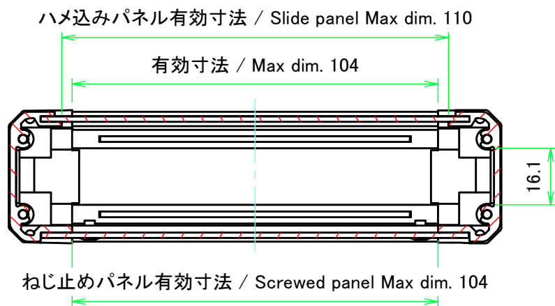
A-A (1:1.5)
