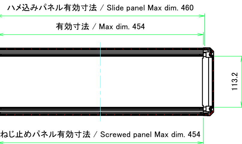
A-A (1:5)
