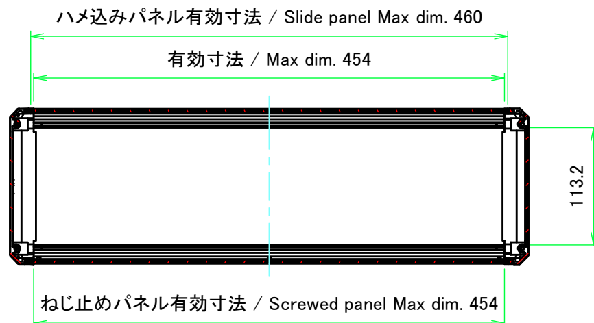
A-A (1:5)
