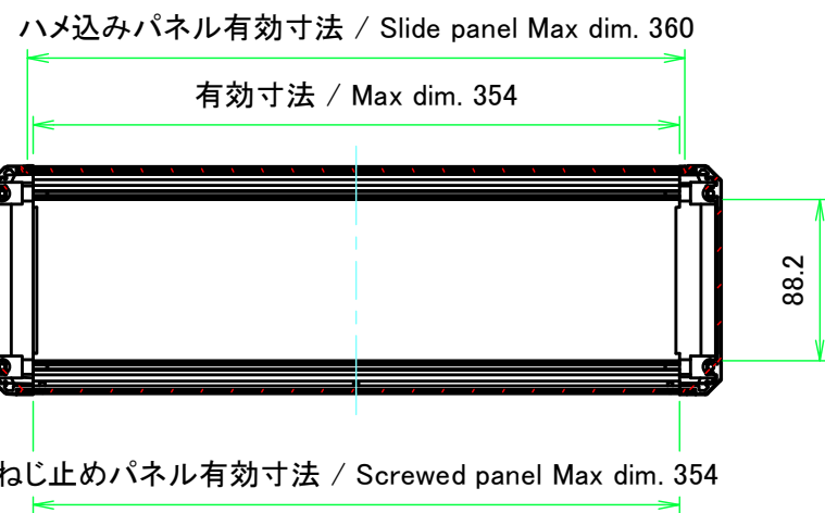
A-A (1:4.5)
