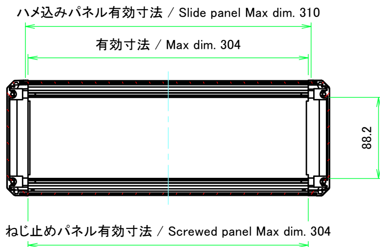
A-A (1:4)
