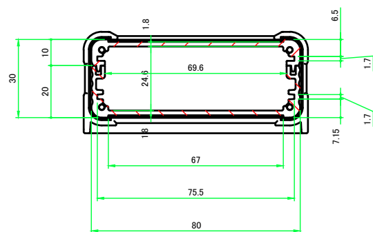
A-A (1:2)
