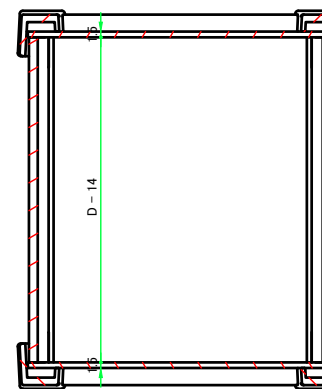
C-C (1:2)
