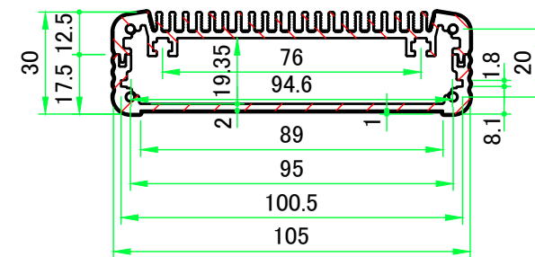
A-A (1:2)
