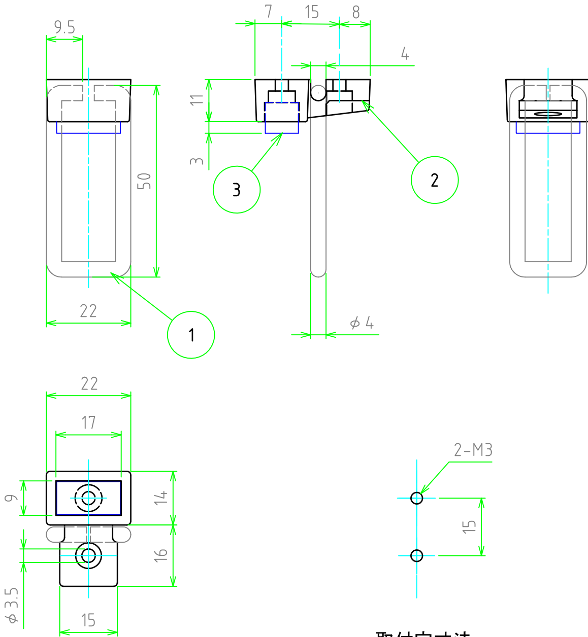
取付穴寸法
