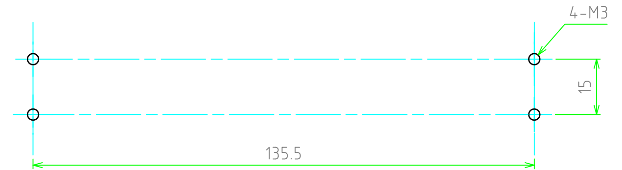
取付穴寸法
