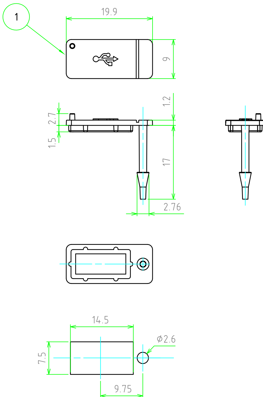
取付穴寸法
