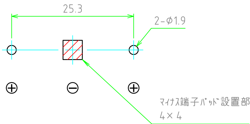
基板実装図
