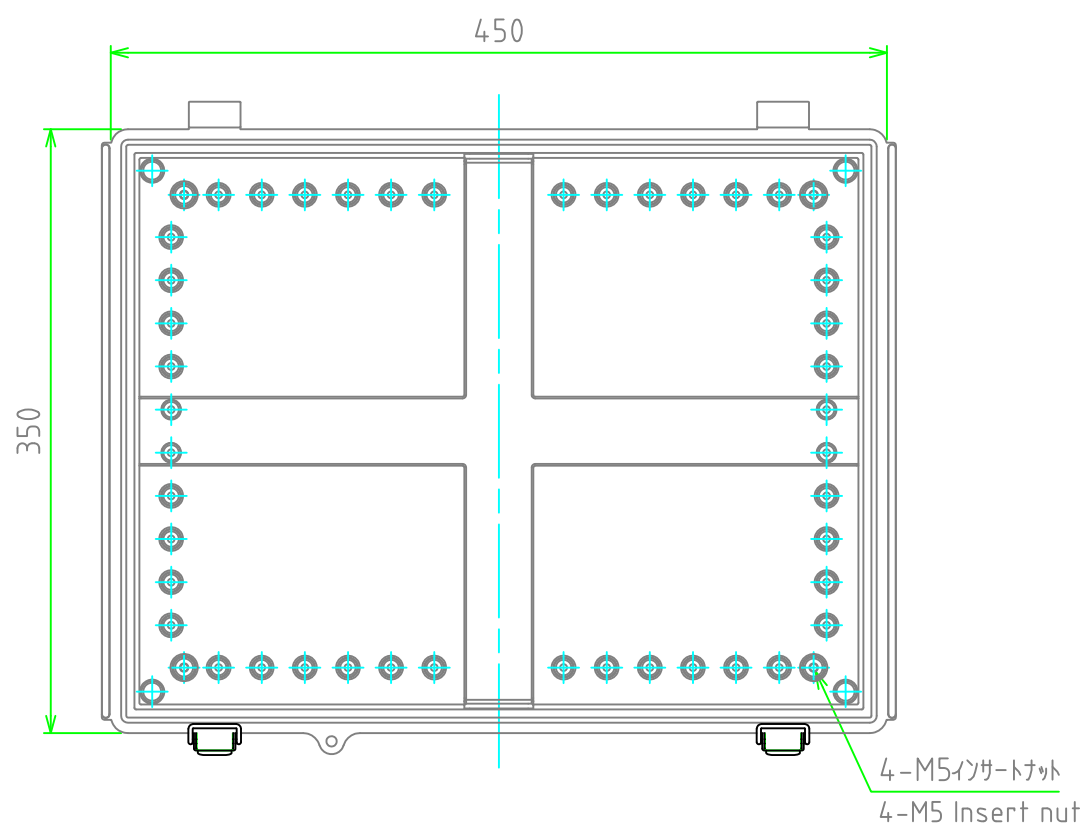
ボディ(内視) Base (Internal View)
