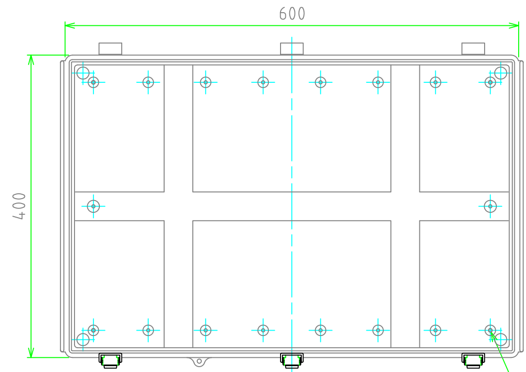
ボディ(内視) Base (Internal View)
