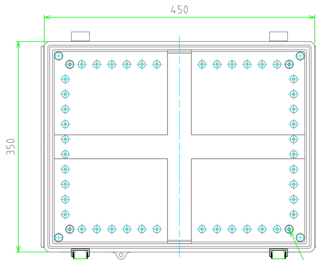
ボディ (内視) Base (Internal View)
