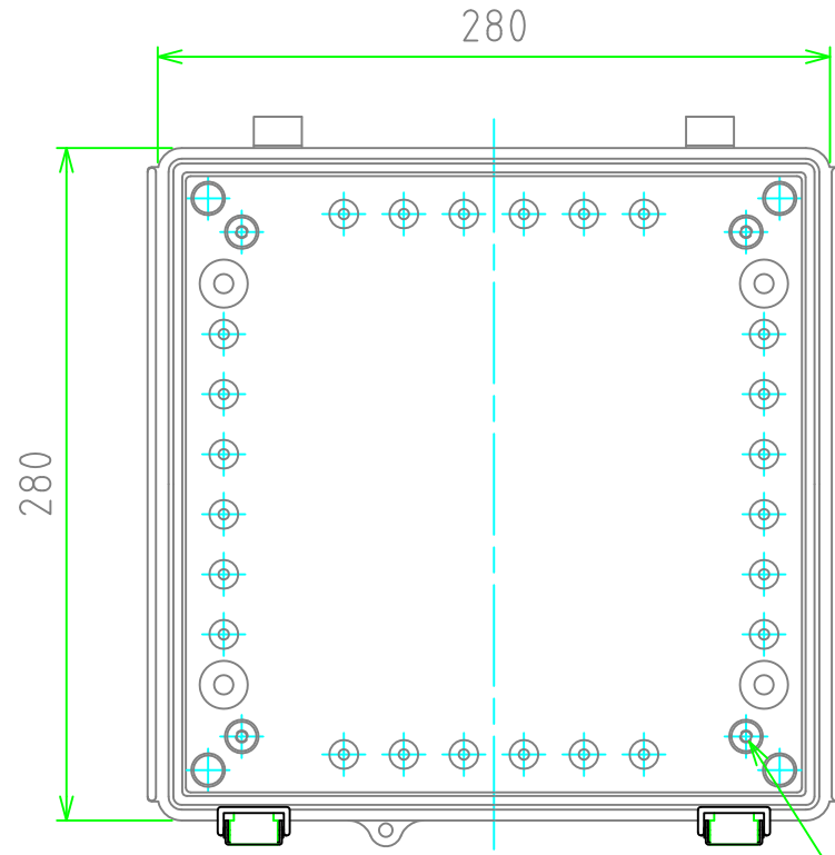
ボディ (内視) Base (Internal View)
