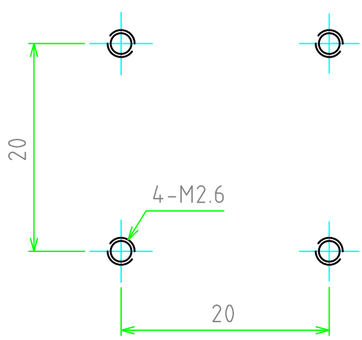
取付穴寸法
